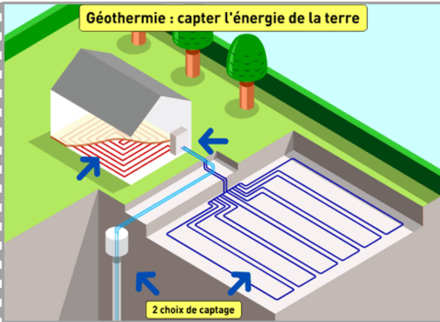
Schéma d'une maison chauffée à l'énergie .....
